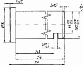
поз 5 М 1:2
