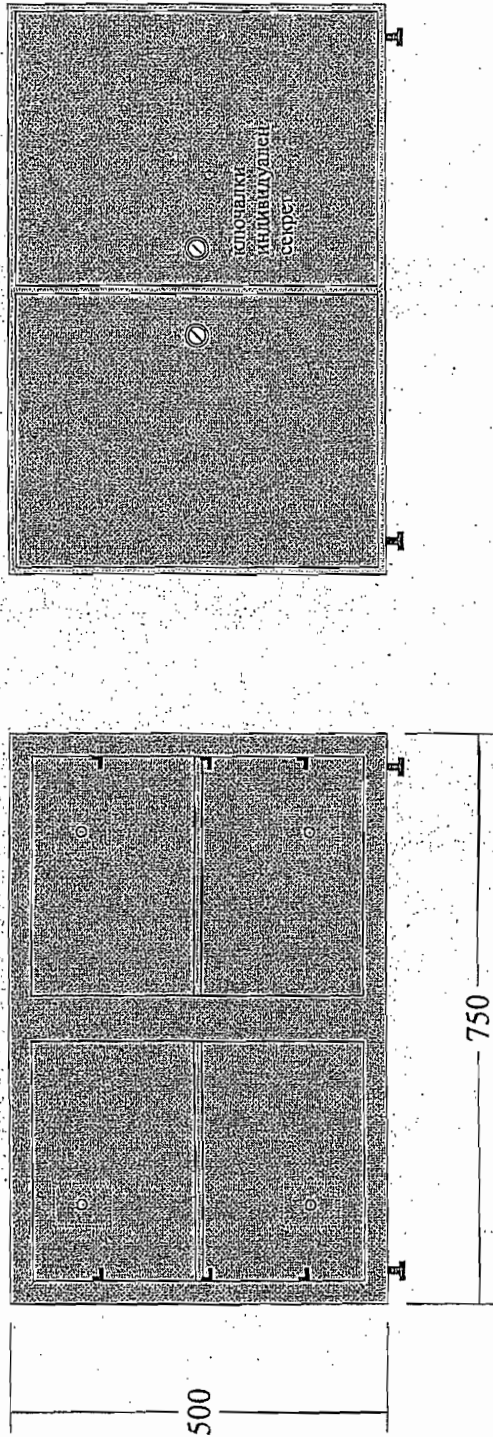
метални планки за монтаж на стена
