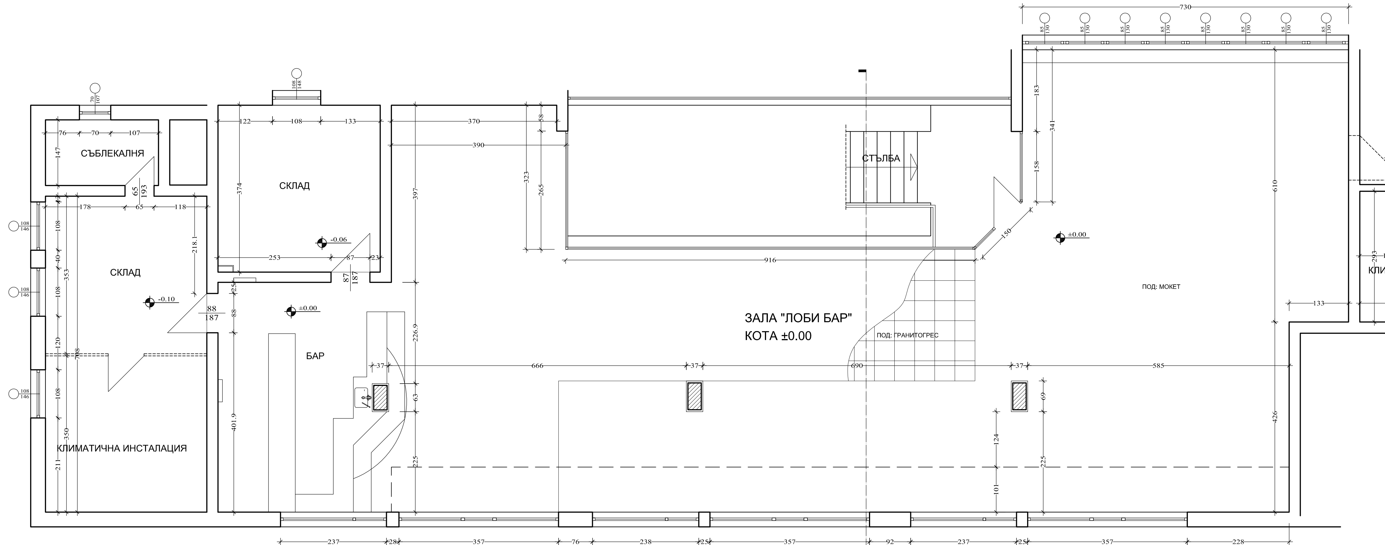
РАЗПРЕДЕЛЕНИЕ КОТА ±0.00 M=1:50 ЗАСЕМАНЕ
