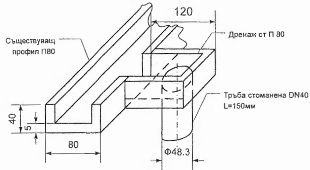
Детайл на дренаж помещения обратни клапи
