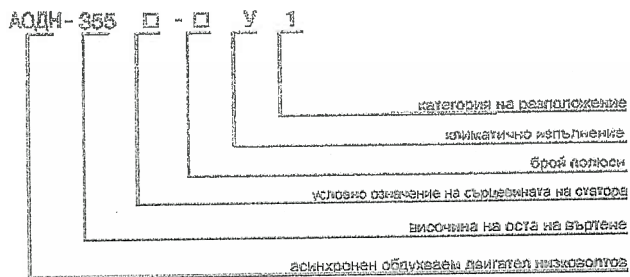
Структура на означението на двигатели тип АОДН
