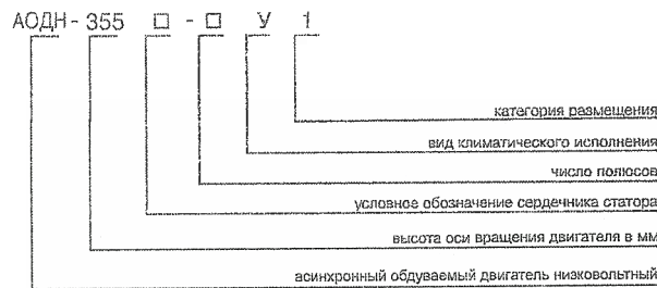
Структура условного обозначения двигателей типа АОДН
