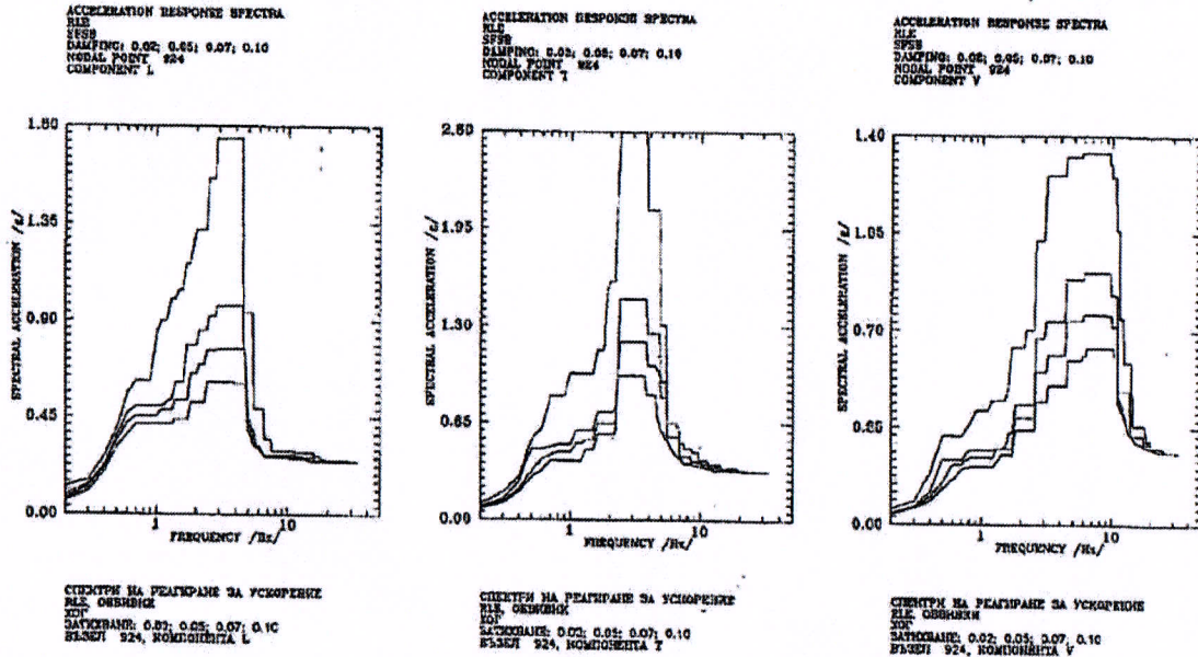
Фиг.Д.25 Спектри на реагиране. Въздействие -RLE. Възед 924
