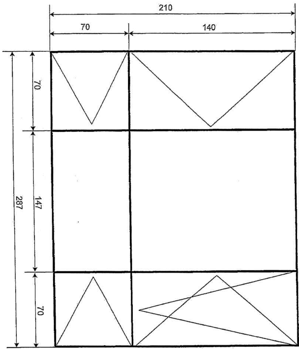
СХЕМА ЗА ИЗРАБОТКА И МОНТАЖ НА ПРОЗОРЕЦ ОТ PVC ДЮГРАМА №1 -- 76p.
