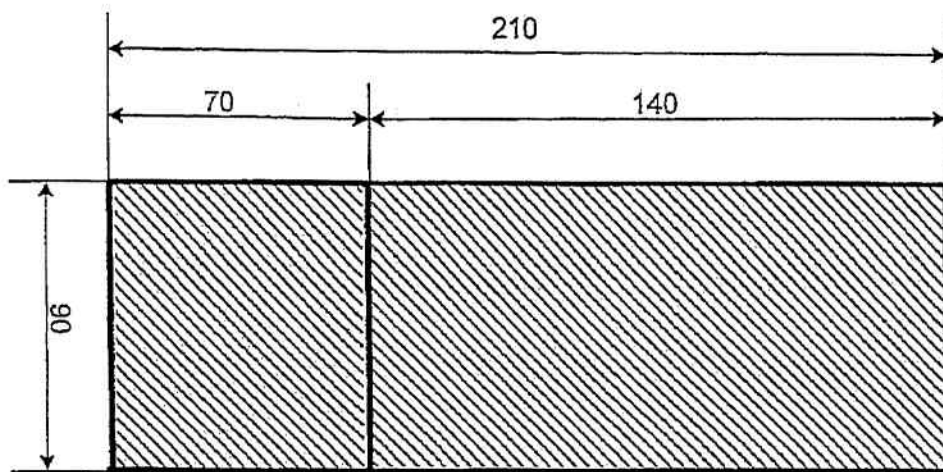
СХЕМА ЗА ИЗРАБОТКА И МОНТАЖ НА БИТОВ ПРОЗОРЕЦ ОТ PVC ДОГРАМА №2 – 16p.
