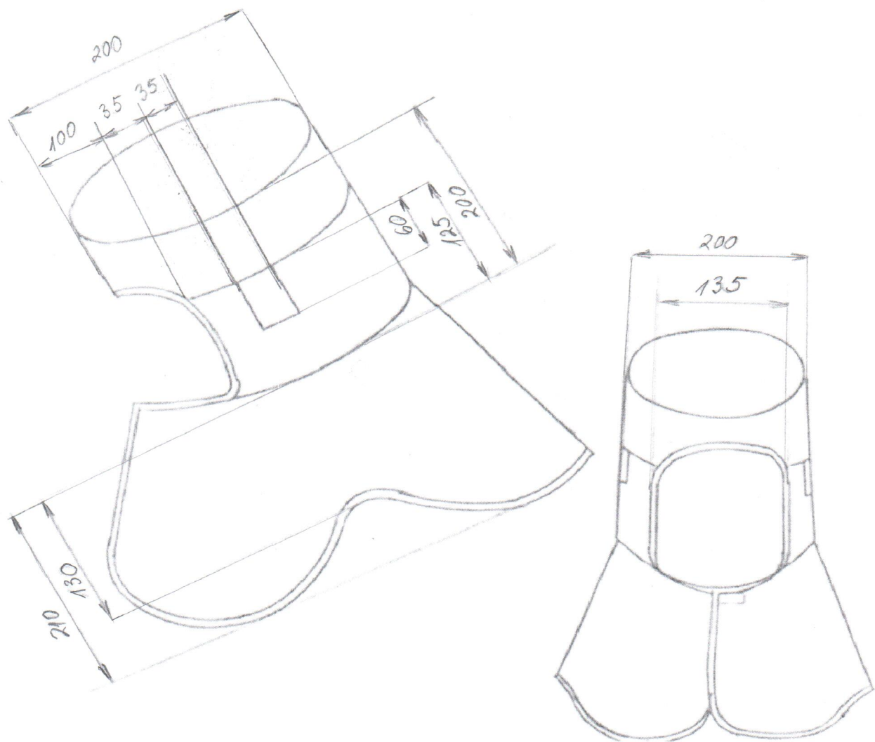
Рис.1 Конструкция и размеры на боне, тип качулка.
