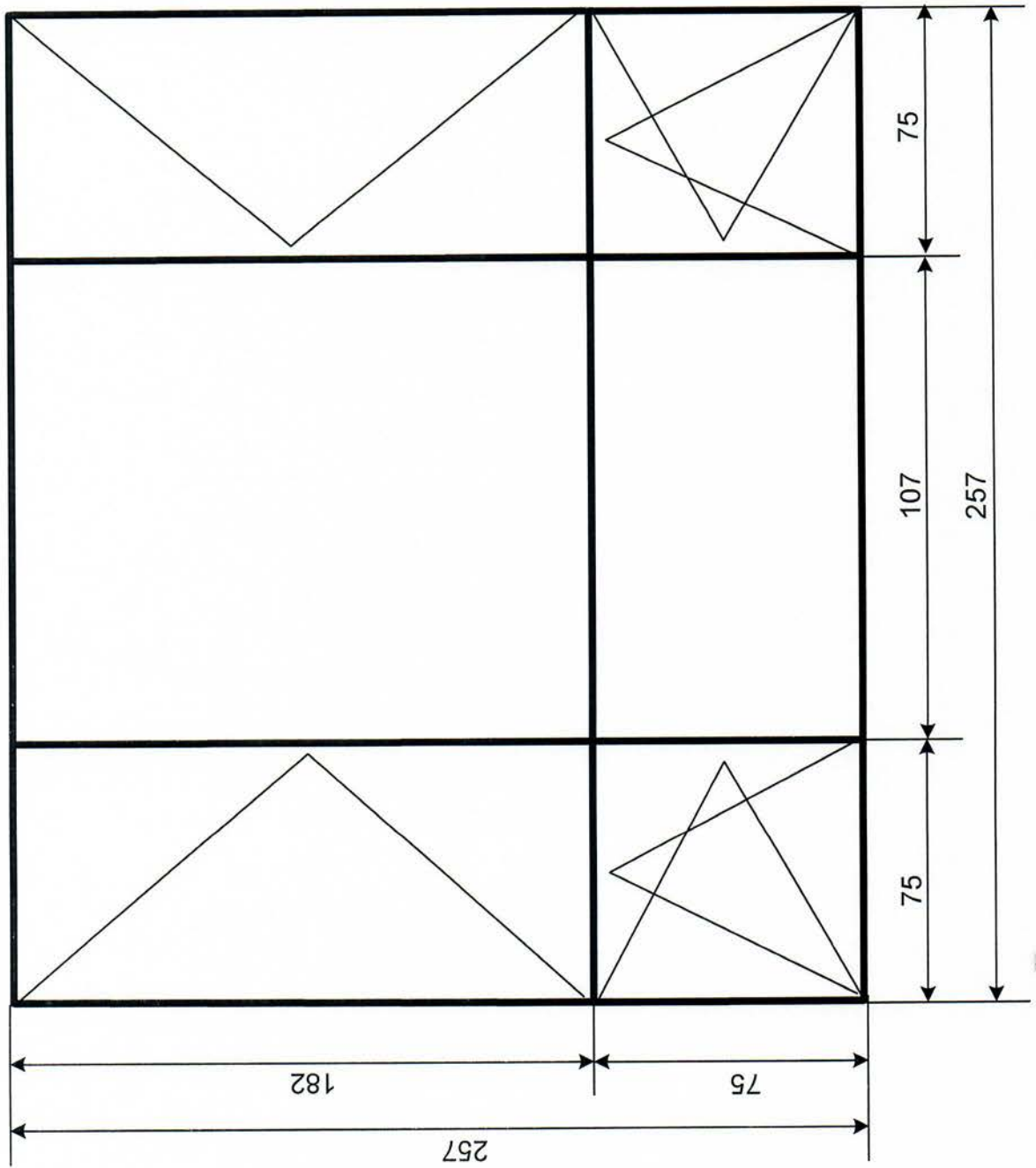
СХЕМА ЗА ИЗРАБОТКА И МОНТАЖ НА ПРОЗОРЕЦ ОТ PVC ДОГРАМА – 5 бр.
