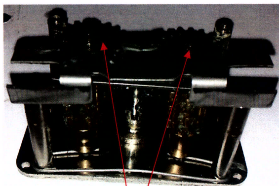
Фигура 2. Износени детайли на блок сигнално - управляващ.
