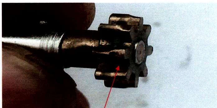
Фигура 2. Износени детайли на блок сигнално - управляващ.
