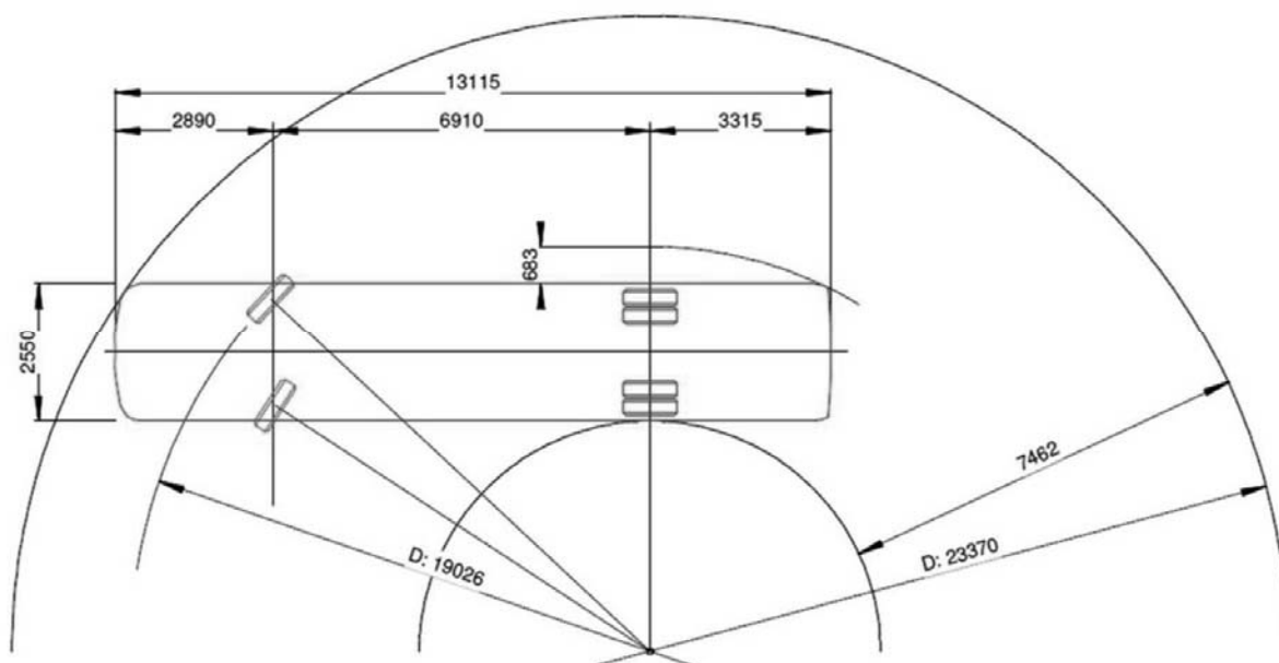
Tourismo 16RHD/2
