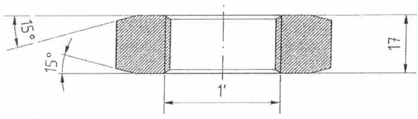
A-A ( 1 : 1 )
