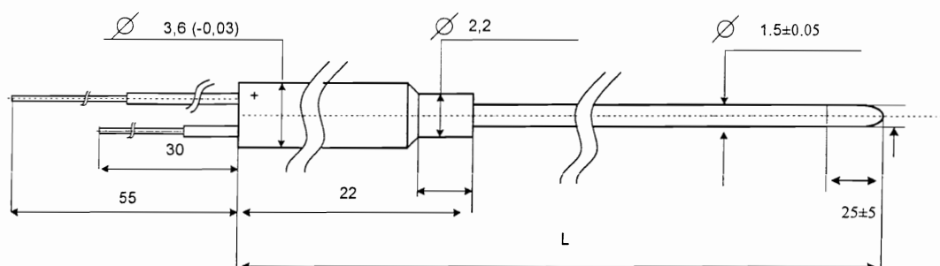
Габаритни размери
