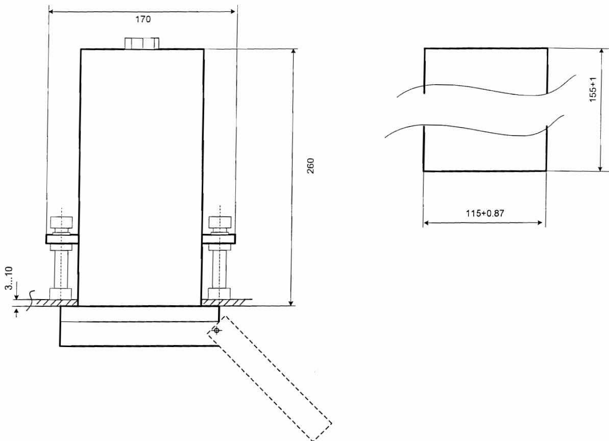
Габаритни размери и размер на монтажния отвор за БП.
