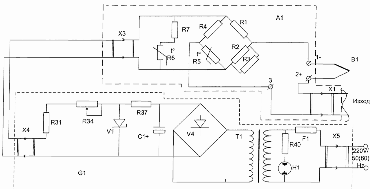
Принципна електрическа схема на канал на УKM-6
