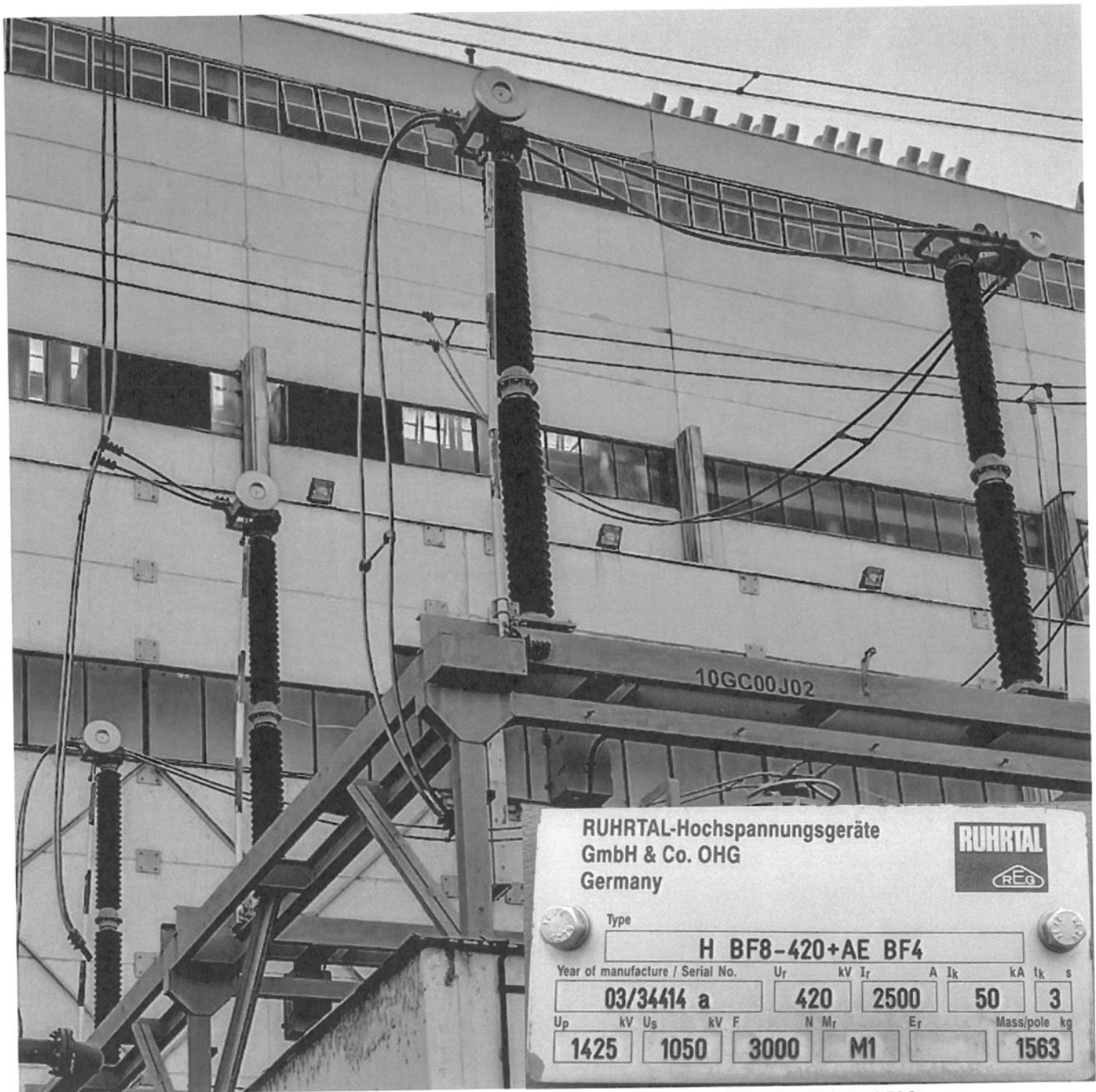
Фиг.2. Външен вид на земен ножов разединител 400kV 10GC00J02, тип: H BF8-420+AE BF4, RUHRTAL – Hochspannungsgerate GmbH & Co. OHG, Germany
