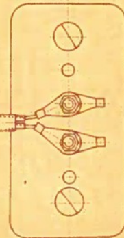
Вид Г на коробку клеммную термообразователи с сопротивлением без крышки
