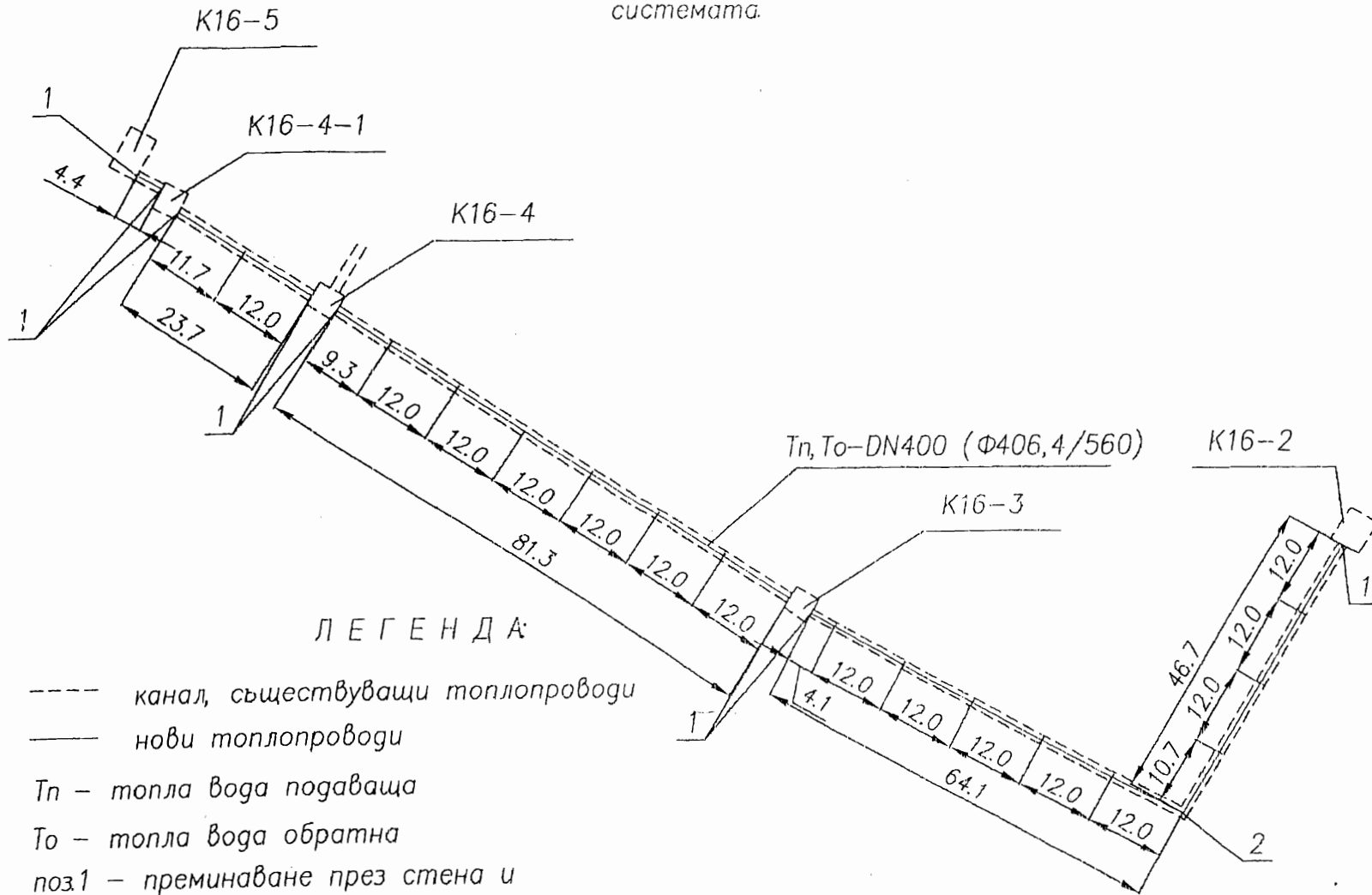
СХЕМА НА ДОСТАВКА НА ТРЪБИ И ЕЛЕМЕНТИ ЗА ТОПЛОПРОВОД УЧАСТЪК 2
