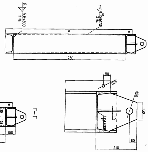
B-B M 1:5
