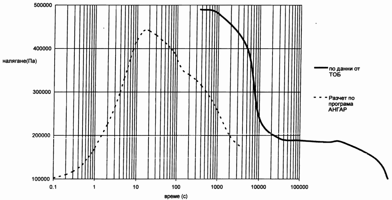
Изменение на налягането в ХО в режим LOCA с разкъсване на ГЦТ
