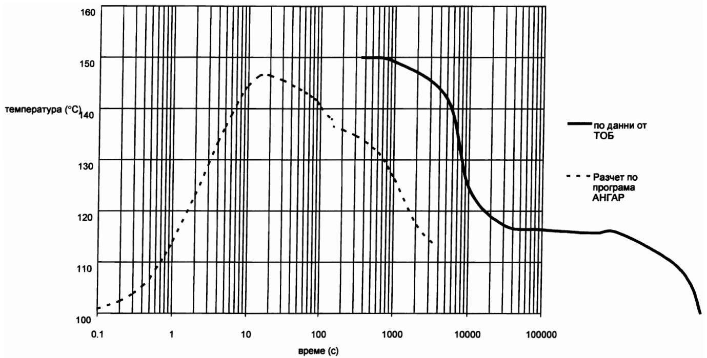
Изменение на температурата на наситената пара в ХО в режим LOCA с разкъсване на ГЦТ
