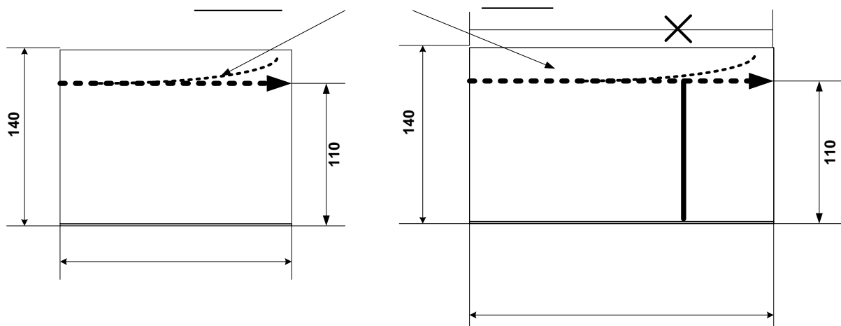
Фигура 2 Разположение на джобовете на защитно облекло (гащеризон)
