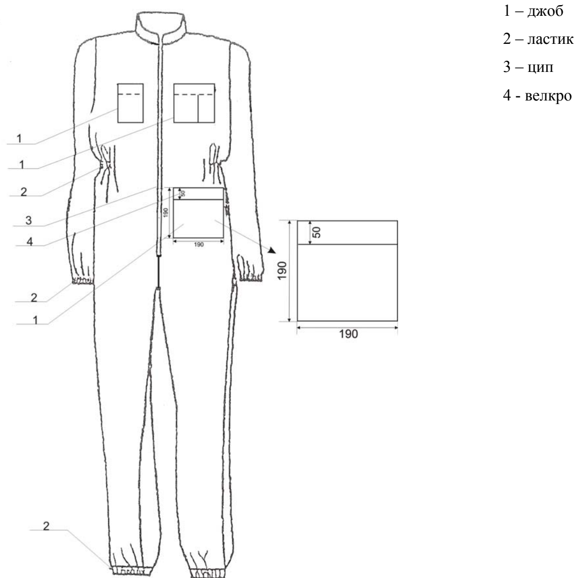
Фигура 1: Защитно облекло(гащеризон) за работа в КЗ
